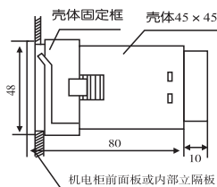
嵌入式安装
