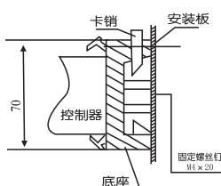
底座式安装
