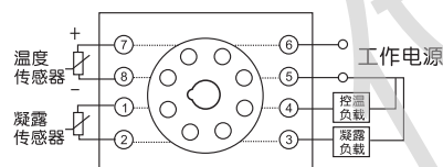
底座式
